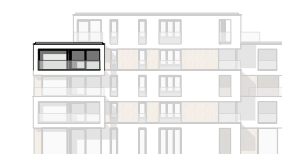
Rechter zijgevel
